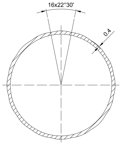
Seccion A-A
