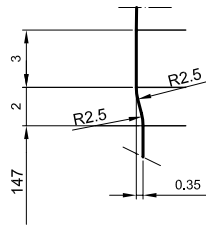
Pormenor A Esc. 5:1
